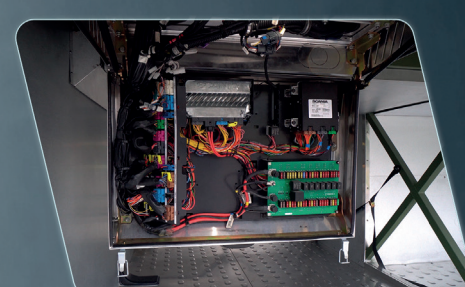
Roteamento de chicotes elétricos otimizado, facilitando manutenção e distribuição dos componentes eletrônicos.
