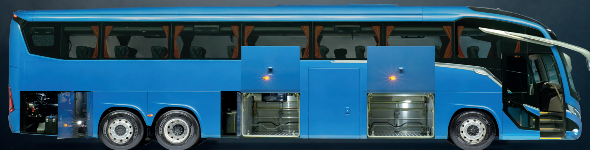
Centrais elétricas padronizadas facilitam a identificação de componentes.
