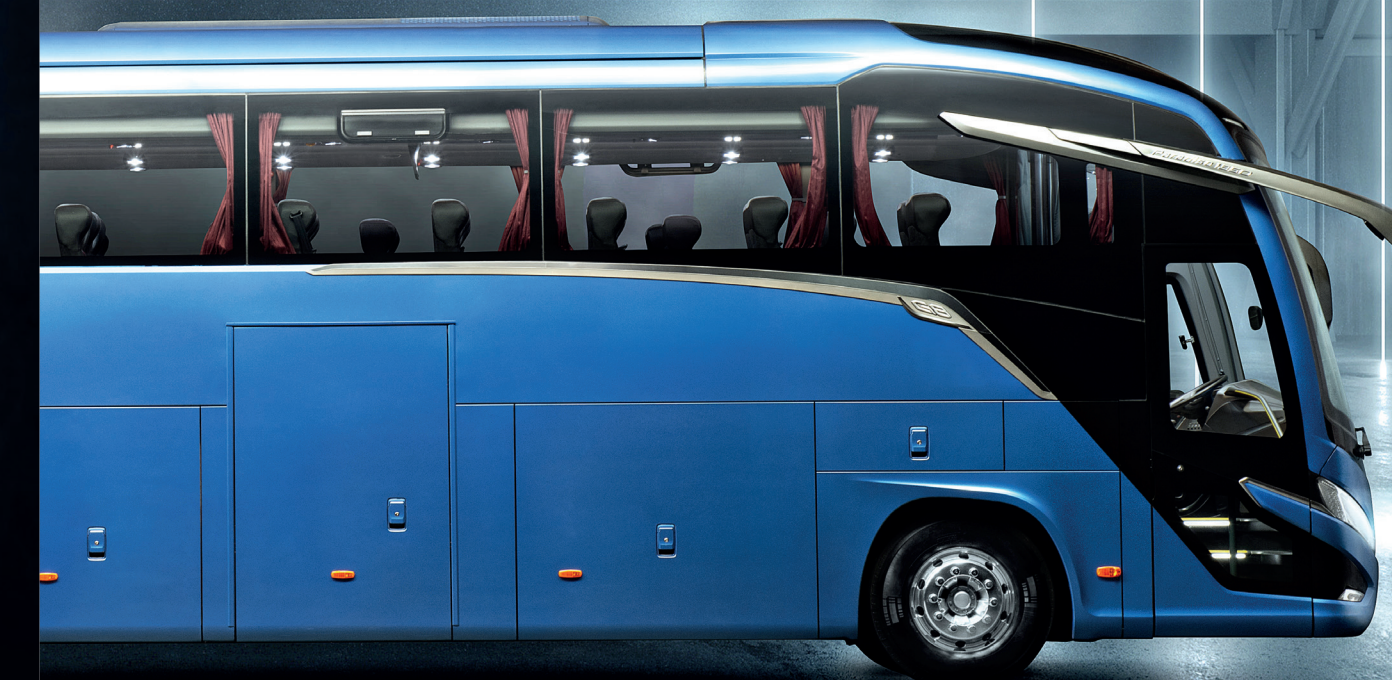
Defroster e ar-condicionado reposicionados para facilitar a manutenção dos equipamentos de refrigeração e aquecimento.
